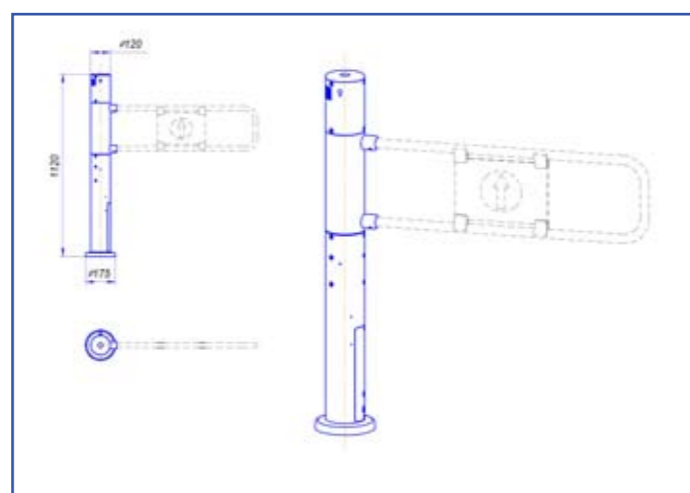
232895000 Portello automatico OverGate - colonna motore - Kit BASE
